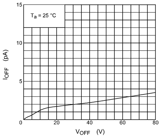
図 12.1.9 I_{OFF} - V_{OFF}
