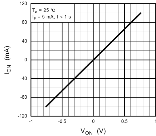
図 12.1.4 I_{ON} - V_{ON}
