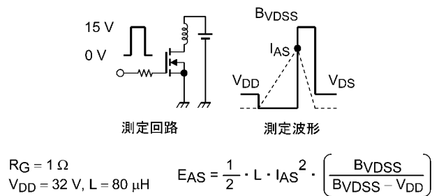
図 8.15 測定回路/測定波形
