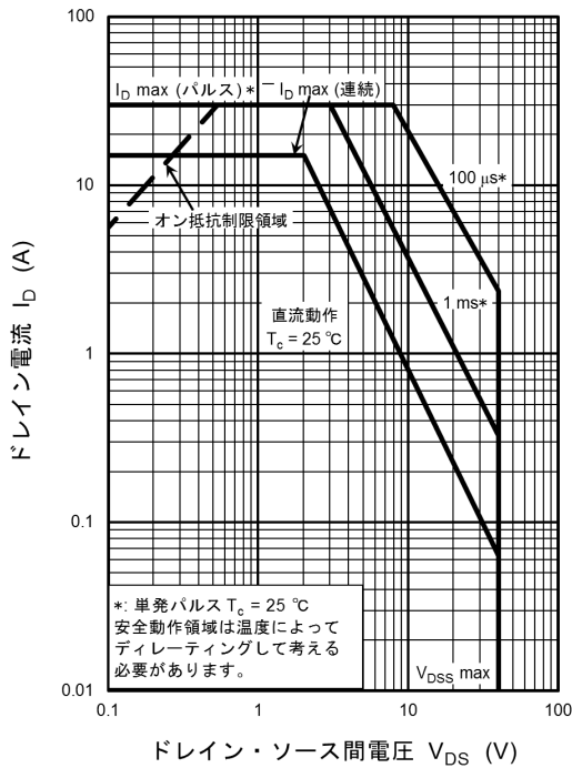
図 8.13 安全動作領域 (最大値 (保証値))
