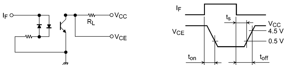
図 10.1 スwitchング時間測定回路, 波形
