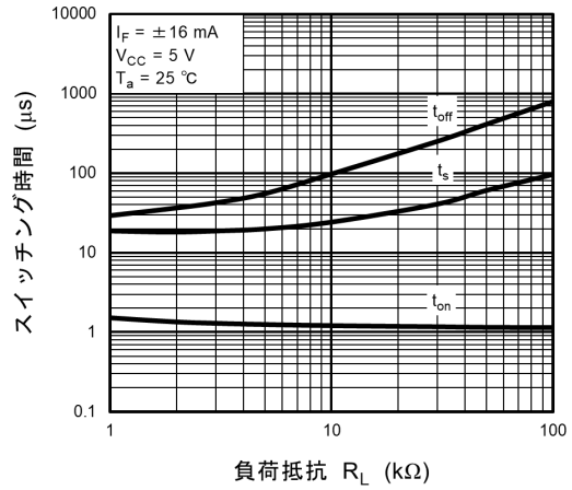
図 11.14 スイッチング時間 - R_L
