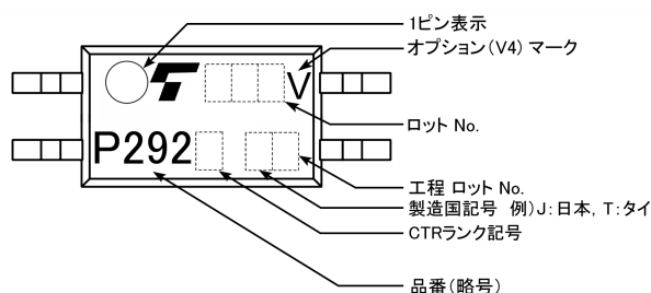
図 15.3 現品表示例 (注)
