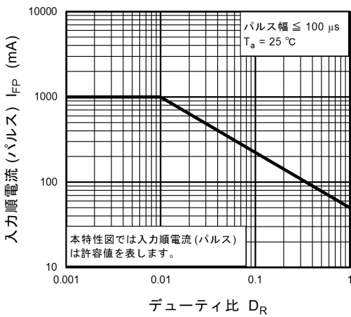
図 11.3 I_{FP} - D_R
