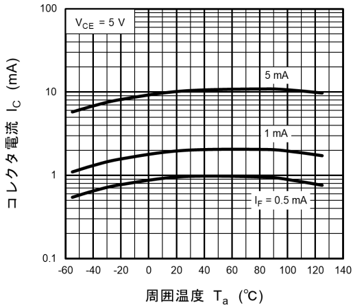
図 11.13 I_C - T_a
