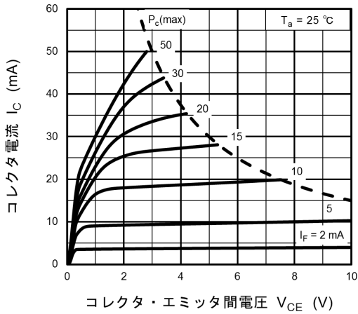
図 11.7 I_C - V_{CE}
