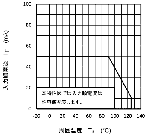
図 11.1 I_F - T_a
