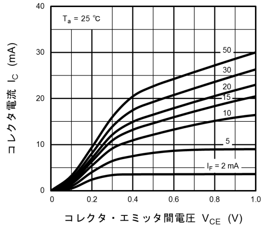
図 11.8 I_C - V_{CE}
