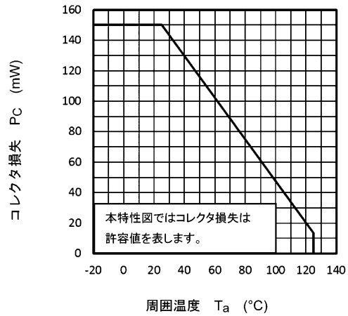
図 11.2 P_C - T_a
