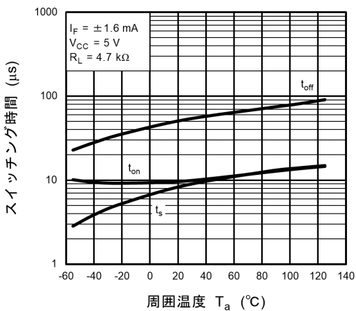
図 11.17 スイッチング時間 - T_a
