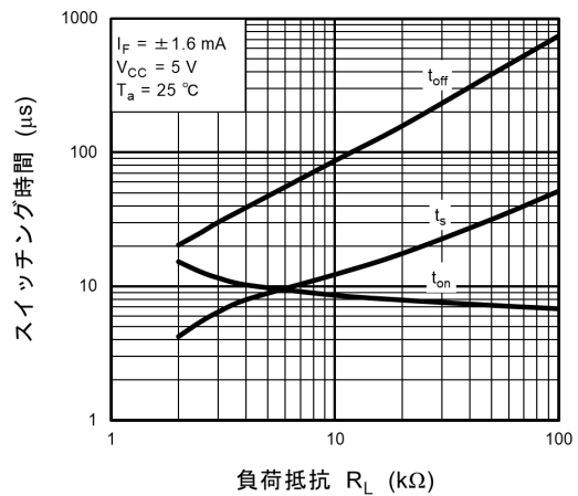
図 11.16 スイッチング時間 - R_L
