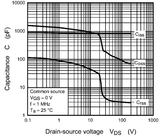
Fig. 8.8 Capacitance - V_{DS}
