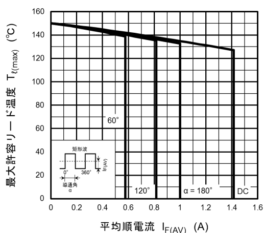
図 10.5 T_{l(max)} - I_{F(AV)}
