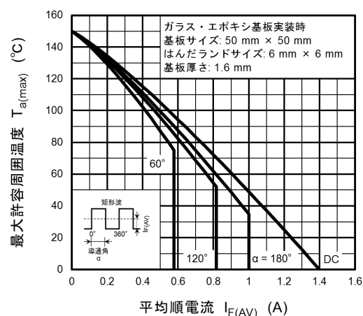
図 10.4 T_{a(max)} - I_{F(AV)}
