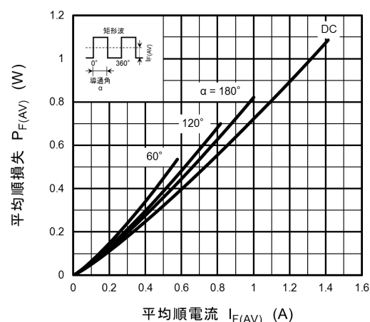
図 10.2 P_{F(AV)} - I_{F(AV)}
