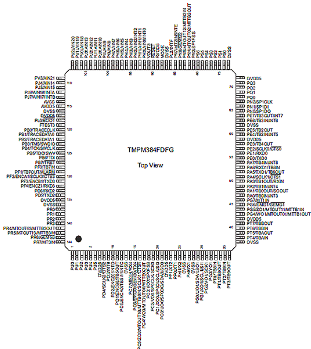
パッケージ: LQFP144 (20 × 20 mm)
