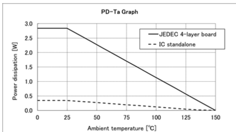
図 7.1 PD-Ta グラフ
