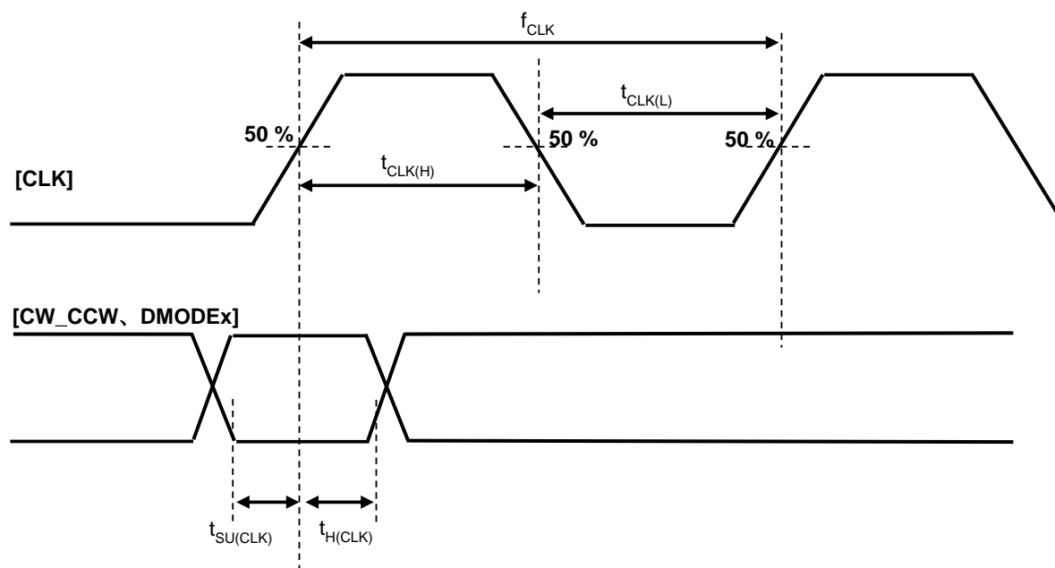
図 9.2 TB67S549FTG(CLK とその他制御信号の関係)
