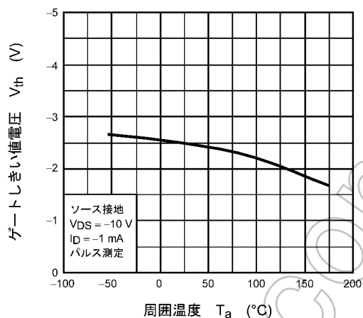
図 8.9 V_{th} - T_a (注8)
