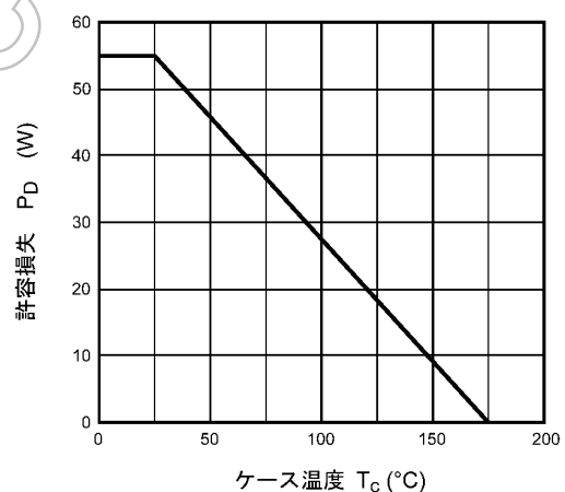
図 8.12 P_D - T_c (注8) (最大値 (保証値))
