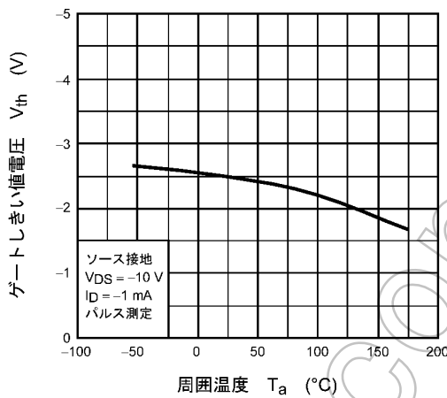
図 8.9 V_{th} - T_a (注8)
