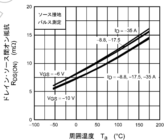
図 8.6 R_{DS(ON)} - T_a (注8)
