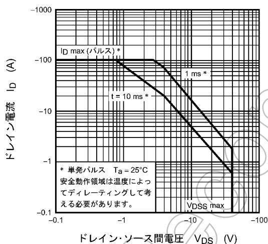
図 8.14 安全動作領域 (最大値 (保証値))
