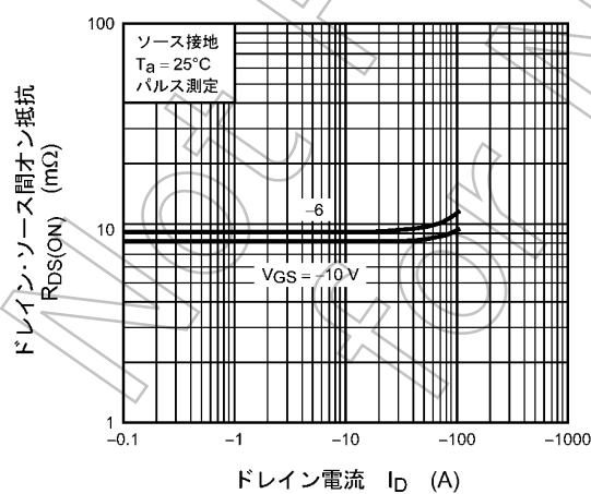
図 8.5 R_{DS(ON)} - I_D
