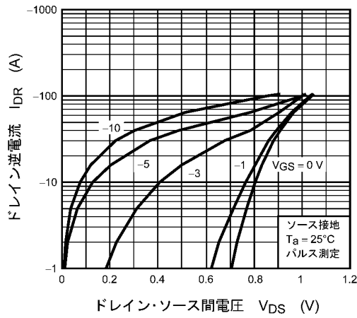
図 8.7 I_{DR} - V_{DS}
