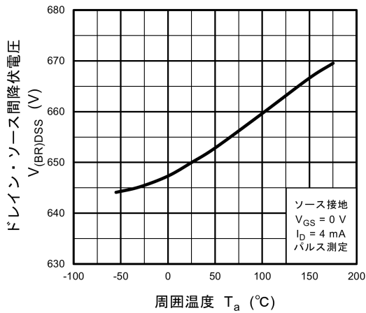
図 8.11 V_{DSS} - T_a
