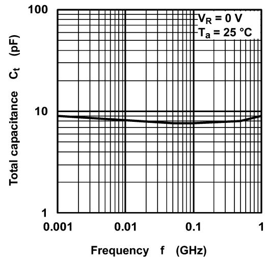
図 8.4 C_t - f
