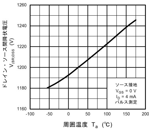
図 8.11 V_{DS} - T_a
