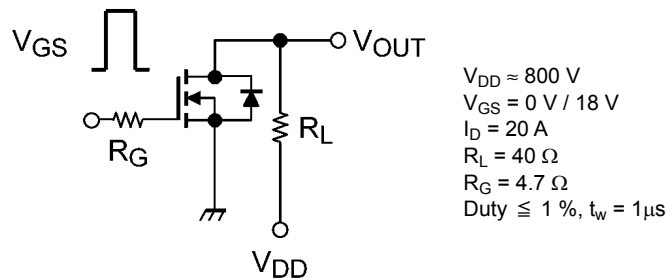
図 6.2.1 スwitching時間の測定回路
