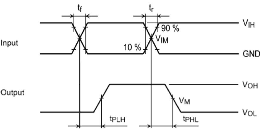
図 9.7.1 t_{PLH} , t_{PHL}
