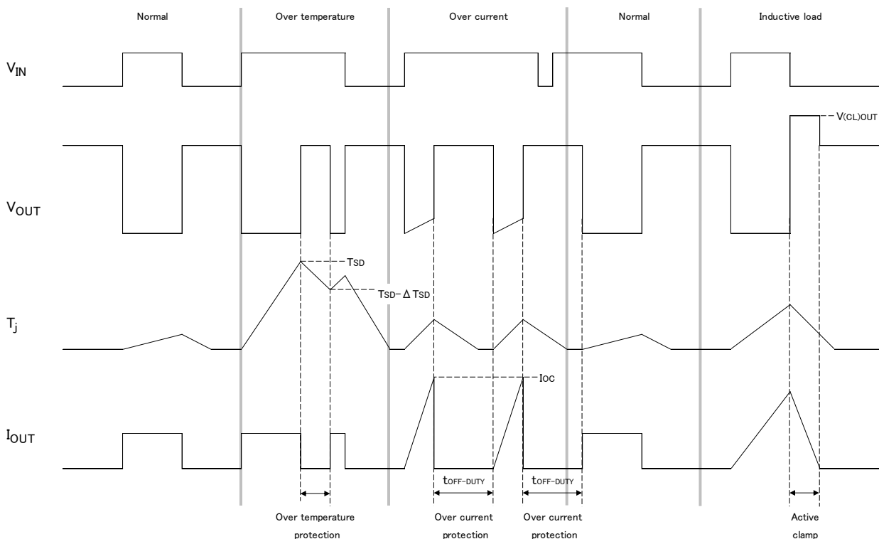
図 7.1 タイミングチャート
