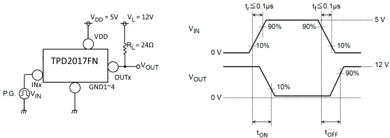
図 11.1 スイッチング時間測定回路
