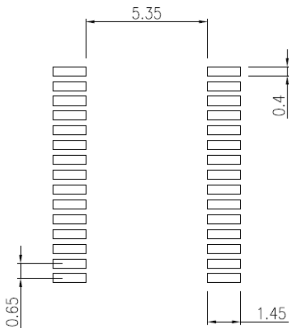
図 13.3 参考ランドパターン
