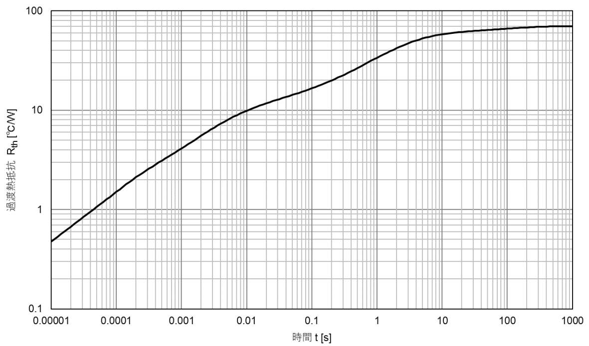
R_{th} - t (1チャンネル動作時)
