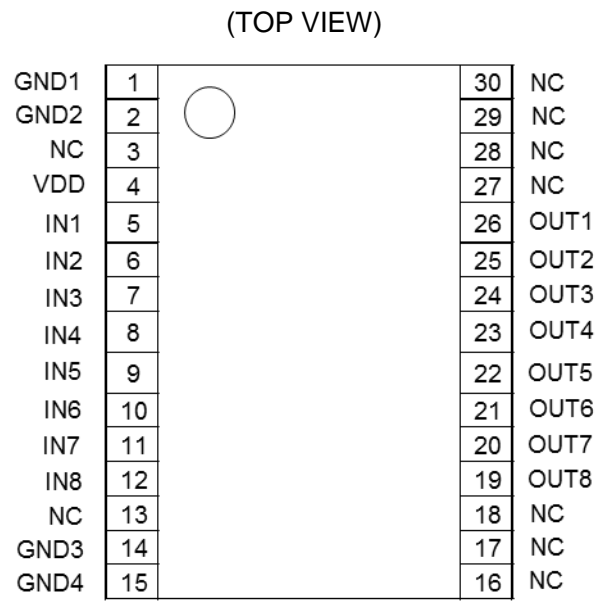
図 5.1 端子配置図
