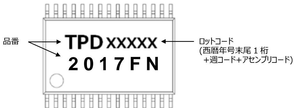
図 13.2 現品表示
