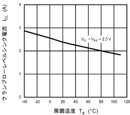
図 13.3.9 I_{CL} - T_a
