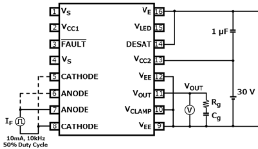
図 13.1.11 t_{pLH} , t_{pHL} , t_r , t_f , |t_{pHL}-t_{pLH}| 測定回路
