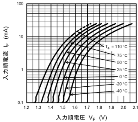
図 13.3.1 I_F - V_F
