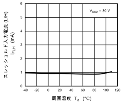
図 13.3.14 I_{FLH} - T_a
