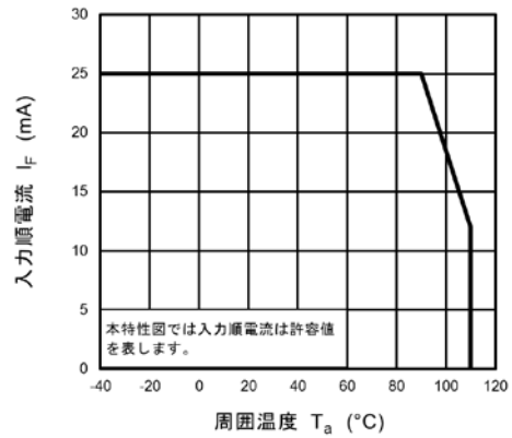
図 13.3.2 I_F - T_a
