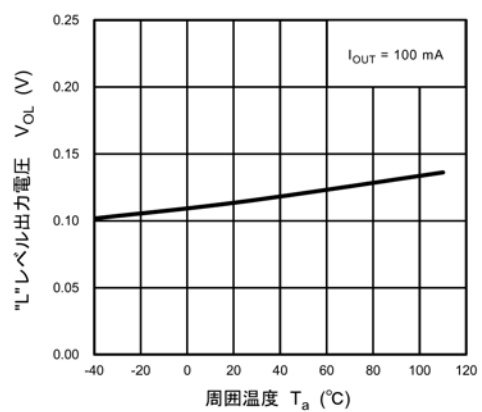
図 13.3.6 V_{OL} - T_a
