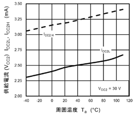
図 13.3.10 I_{CC2} - T_a
