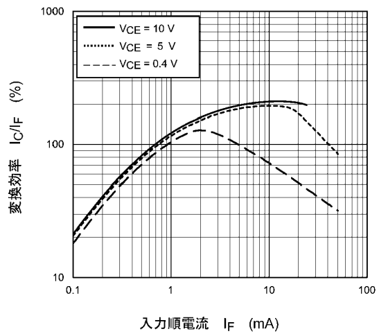
図 11.12 I_C/I_F - I_F
