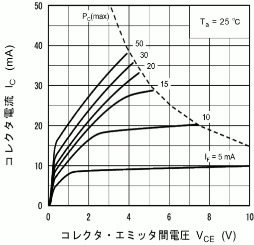
図 11.7 I_C - V_{CEO}
