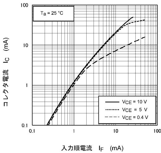
図 11.11 I_C - I_F
