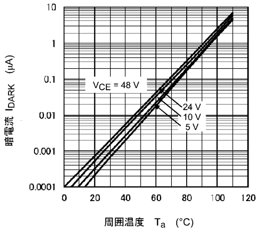
図 11.9 I_{\text{DARK}} - T_a
