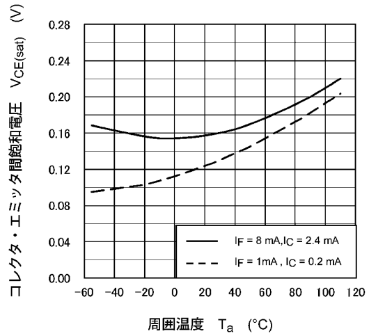
図 11.10 V_{CE(\text{sat})} - T_a
