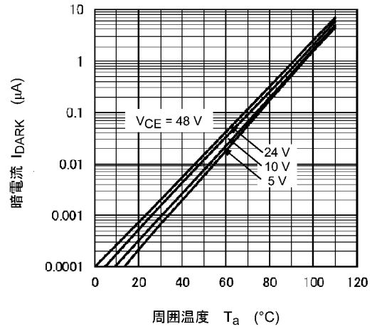
図 11.10 I_{\text{DARK}} - T_a
