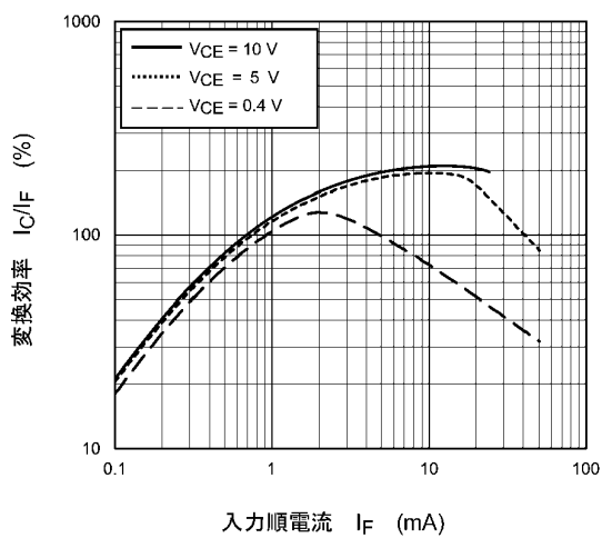
図 11.11 I_C/I_F - I_F
