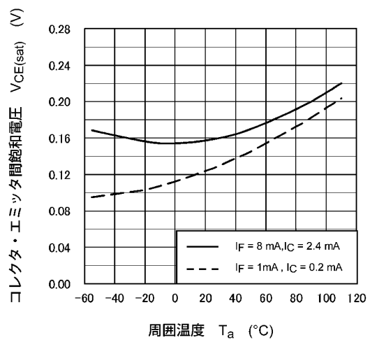
図 11.12 V_{CE(\text{sat})} - T_a
