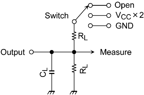
AC電気的特性測定回路
