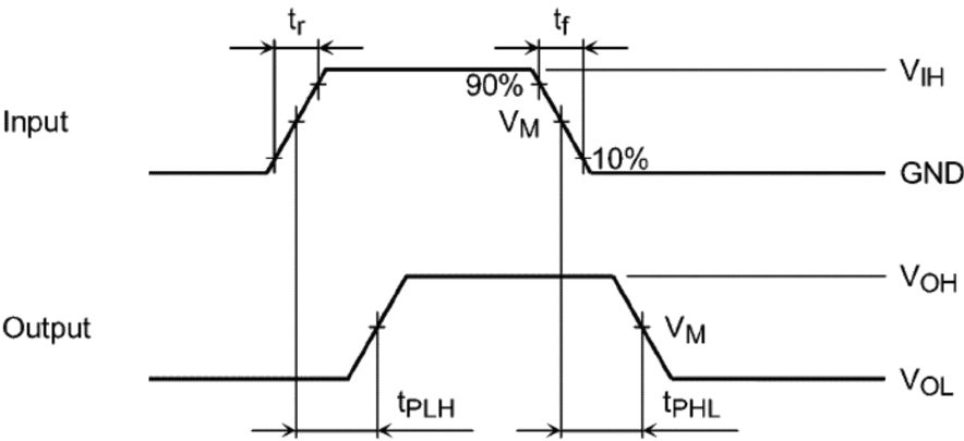
図 9.8.1 t_{PLH} , t_{PHL}
