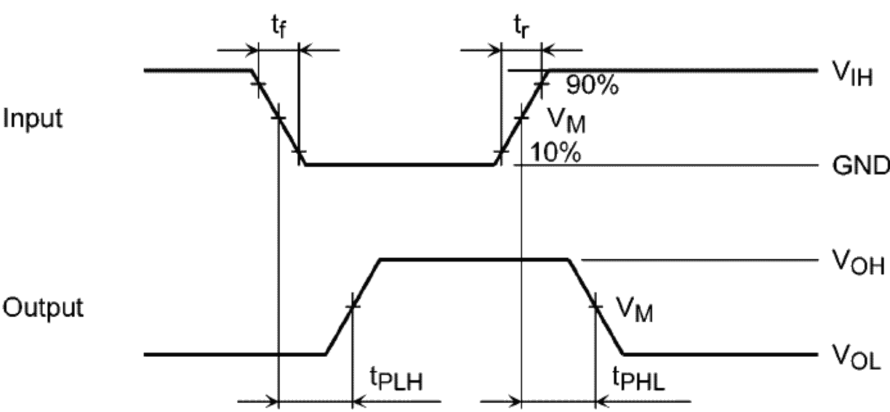
図 9.7.1 t_{PLH} , t_{PHL}
