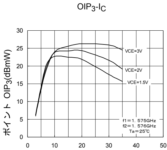
3次相互変調歪出カインターセプト
