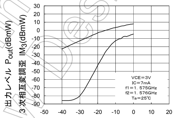
P_{\text{out}}, \text{IM}_3\text{-}P_{\text{in}}
