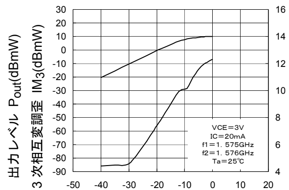
P_{\text{out}}, \text{IM}_3\text{-}P_{\text{in}}
