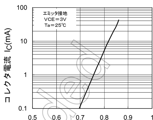
I_C-V_{BE}
