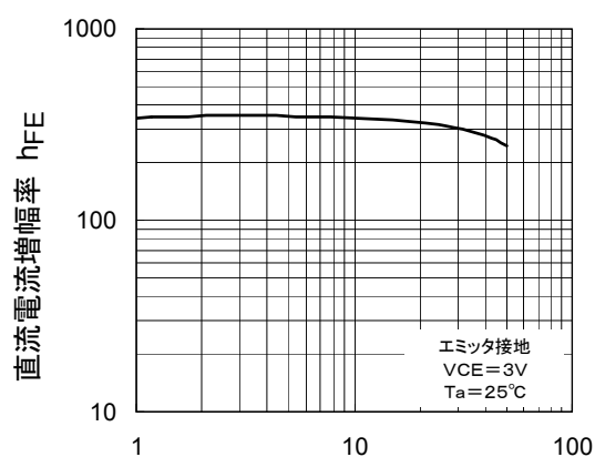
h_{FE}-I_C
