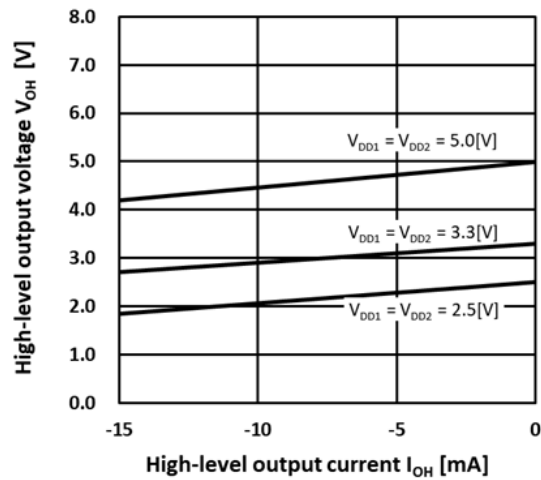
Fig.13.7. V_{OH} - I_{OH}
