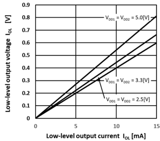
Fig.13.8. V_{OL} - I_{OL}
