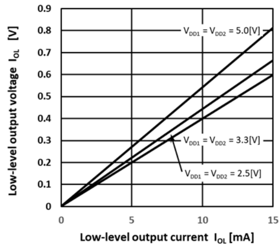
Fig.13.8. V_{OL} - I_{OL}
