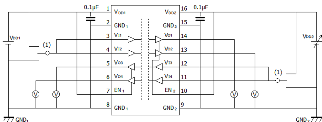
Fig.12.1.9. DCL542L01/DCL542H01 VDD2UV+/ VDD2UV-Test Circuit
