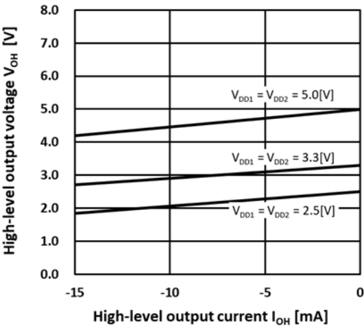
図 13.7. V_{OH}-I_{OH}
