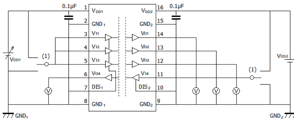
図 12.1.5. DCL541A01/DCL541B01 V_{DD1UV+}/V_{DD1UV-} 特性測定回路図
