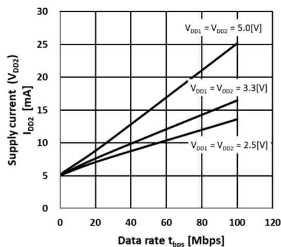
図 13.2. DCL540x01 I_{DD2} 動作電流—データレート
