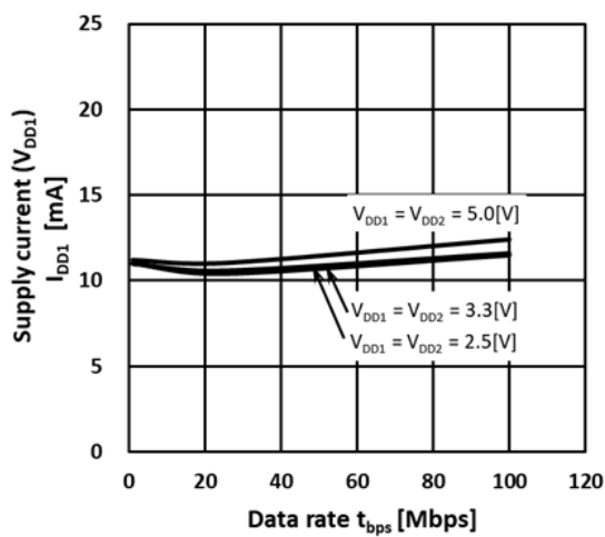
図 13.1. DCL540x01 I_{DD1} 動作電流—データレート
