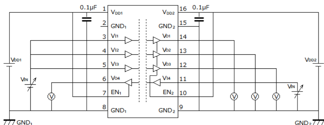
図 12.3.3. DCL541L01/DCL541H01 V_{IH}/V_{IL} 特性測定回路図
