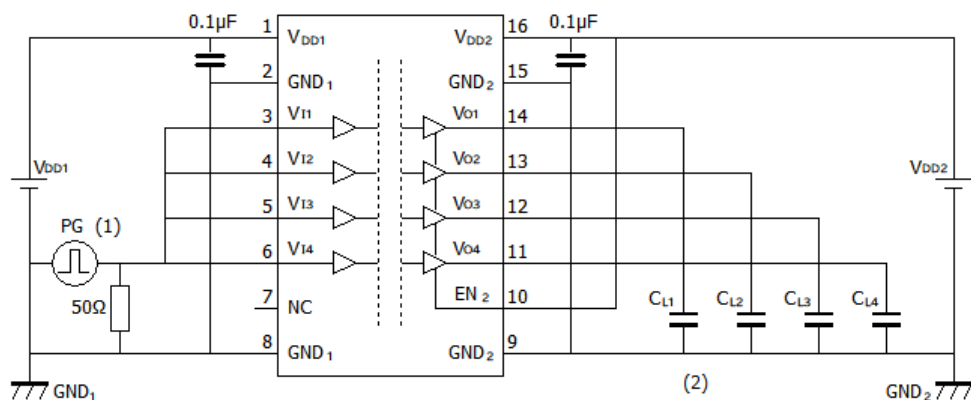
図 12.4.1. DCL540C01/DCL540D01 Switching 特性測定回路図
