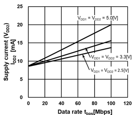
図 13.6. DCL542x01 I_{DD2} 動作電流—データレート
