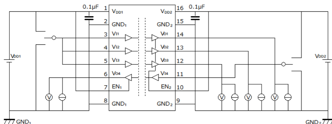
図 12.2.3. DCL541L01/DCL541H01 V_{OH}/V_{OL} 特性測定回路図
