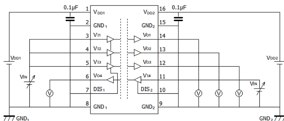
図 12.3.5. DCL541A01/DCL541B01 V_{IH}/V_{IL} 特性測定回路図
