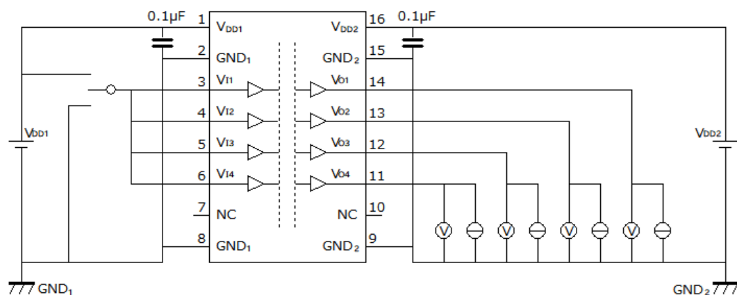
図 12.2.1. DCL540C01/DCL540D01 V_{OH}/V_{OL} 特性測定回路図
