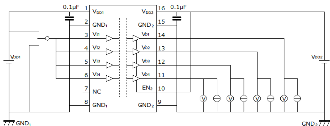
図 12.2.2. DCL540L01/DCL540H01 V_{OH}/V_{OL} 特性測定回路図
