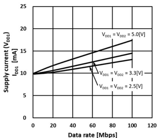
図 13.3. DCL541x01 I_{DD1} 動作電流—データレート
