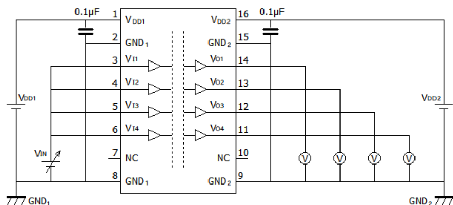
図 12.3.1. DCL540C01/DCL540D01 V_{IH}/V_{IL} 特性測定回路図
