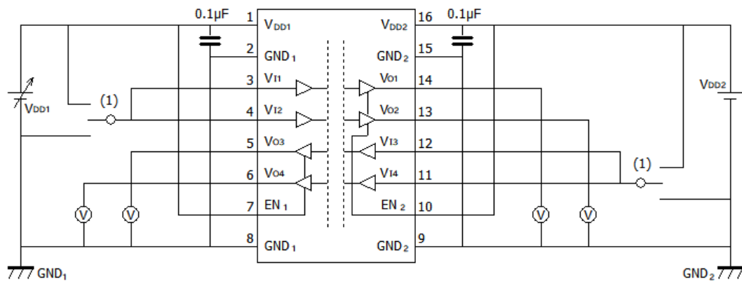
図 12.1.4. DCL542L01/DCL542H01 V_{DD1UV+}/V_{DD1UV-} 特性測定回路図
