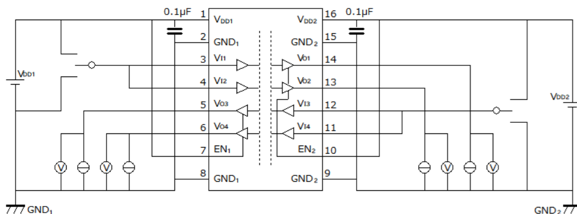
図 12.2.4. DCL542L01/DCL542H01 V_{OH}/V_{OL} 特性測定回路図
