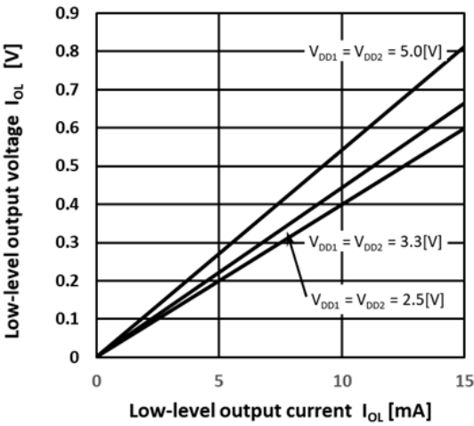
図 13.8. V_{OL}-I_{OL}
