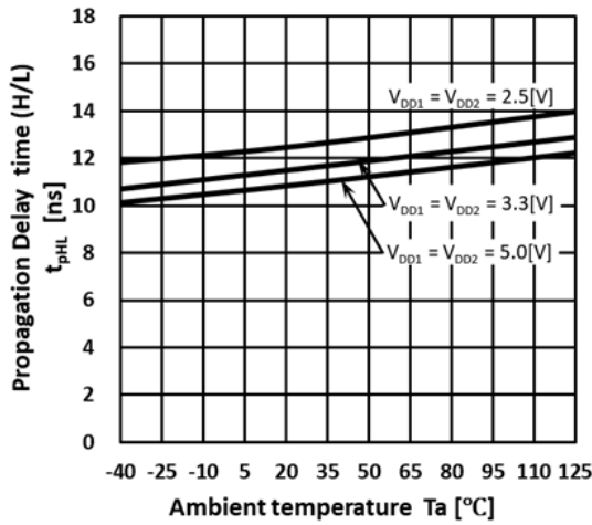
図 13.10. 伝搬遅延 t_{PLH}-T_a
