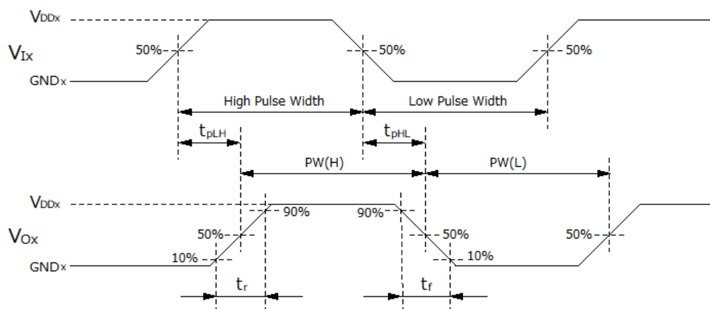
図 12.4.6. DCL54xx01 Switching 特性波形図
