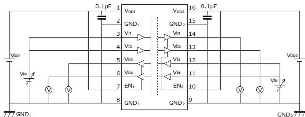
図 12.3.4. DCL542L01/DCL542H01 V_{IH}/V_{IL} 特性測定回路図
