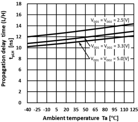
図 13.9. 伝搬遅延 t_{PLH}-T_a
