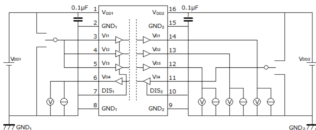
図 12.2.5. DCL541A01/DCL541B01 V_{OH}/V_{OL} 特性測定回路図
