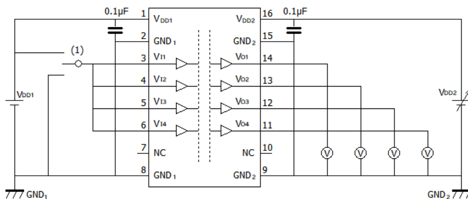
図 12.1.6. DCL540C01/DCL540D01 V_{DD2UV+}/V_{DD2UV-} 特性測定回路図
