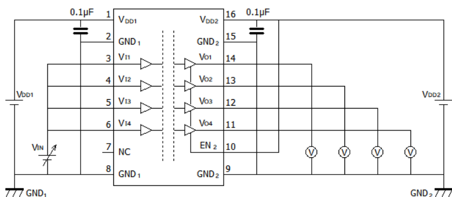
図 12.3.2. DCL540L01/DCL540H01 V_{IH}/V_{IL} 特性測定回路図
