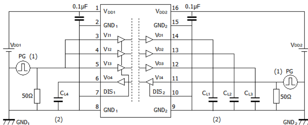
図 12.4.4. DCL542L01/DCL542H01 Switching 特性測定回路図
