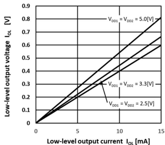
図 13.8. V_{OL}-I_{OL}
