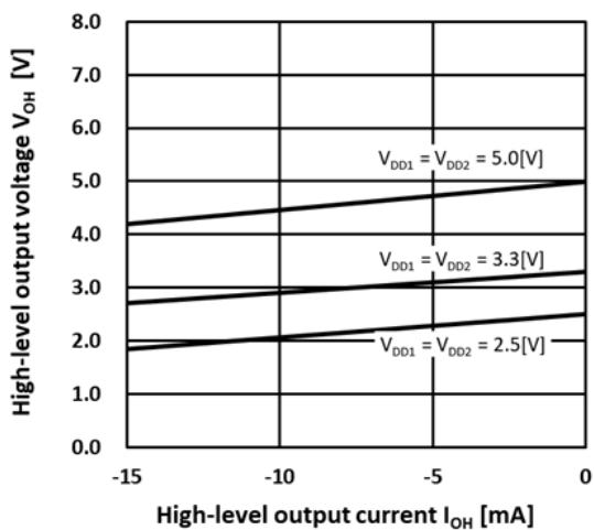
図 13.7. V_{OH}-I_{OH}
