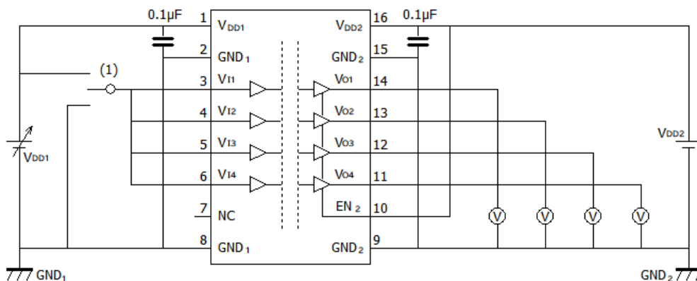
図 12.1.2. DCL540L01/DCL540H01 V DD1UV+ / V DD1UV- 特性測定回路図
