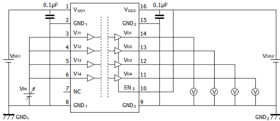
图 12.3.2. DCL540L01/DCL540H01 V_{IH}/V_{IL} 特性測定回路図
