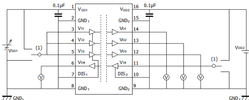
図 12.1.3. DCL541A01/DCL541B01 V DD1UV+ / V DD1UV- 特性測定回路図
