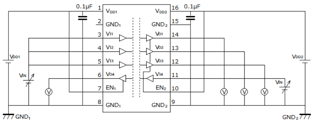
图 12.3.3. DCL541L01/DCL541H01 V_{IH}/V_{IL} 特性測定回路図
