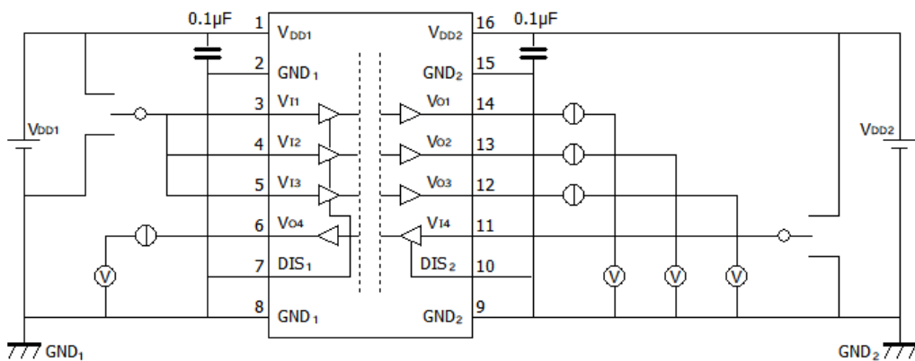
图 12.2.3. DCL541A01/DCL541B01 V_{OH}/V_{OL} 特性测定回路图
