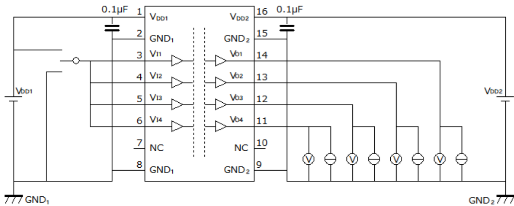
图 12.2.1. DCL540C01/DCL540D01 V_{OH}/V_{OL} 特性測定回路図
