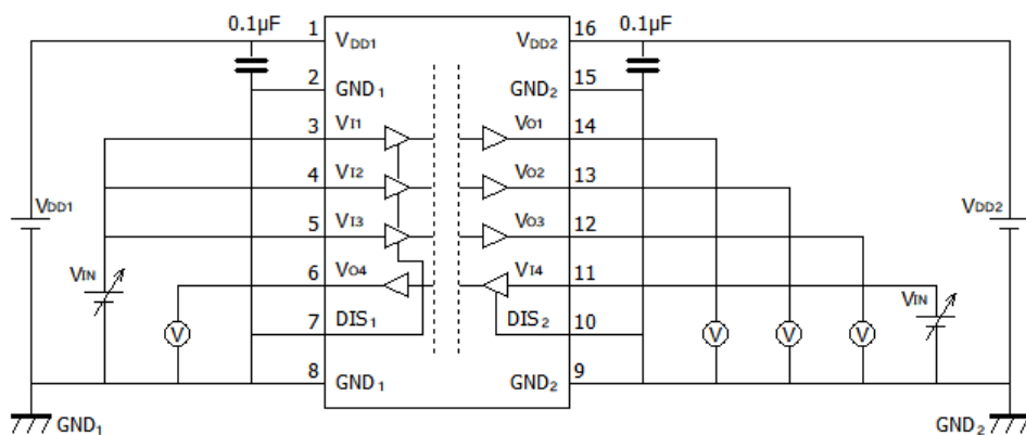
图 12.3.3. DCL541A01/DCL541B01 V_{IH}/V_{IL} 特性測定回路図
