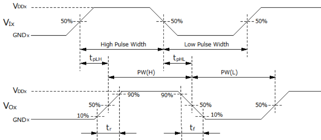
図 12.4.1. DCL540C01/DCL540D01 Switching 特性測定回路図と波形図
