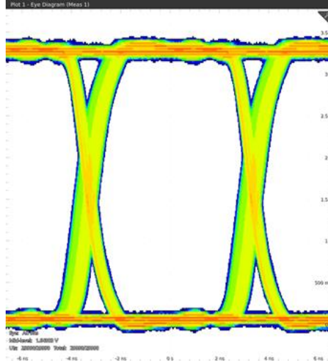
図14.1 DCL541A01のアイ・ダイアグラム例
