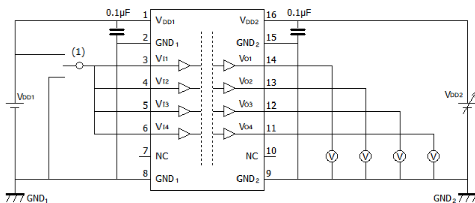
图 12.1.6. DCL540C01/DCL540D01 V_{DD2U+}/V_{DD2U-} 特性测定回路图
