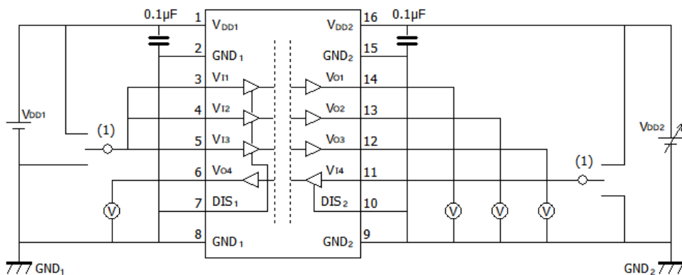
图 12.1.6. DCL541A01/DCL541B01 V DD2UV+ / V DD2UV- 特性测定回路图
