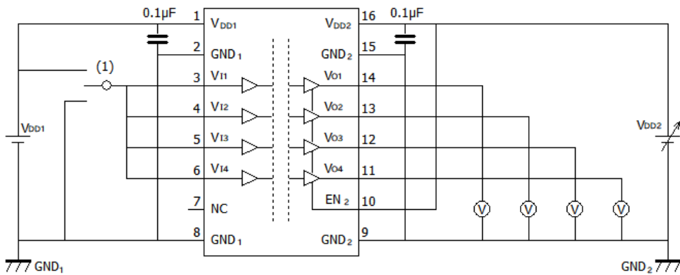
图 12.1.5. DCL540L01/DCL540H01 V DD2UV+ / V DD2UV- 特性测定回路图
