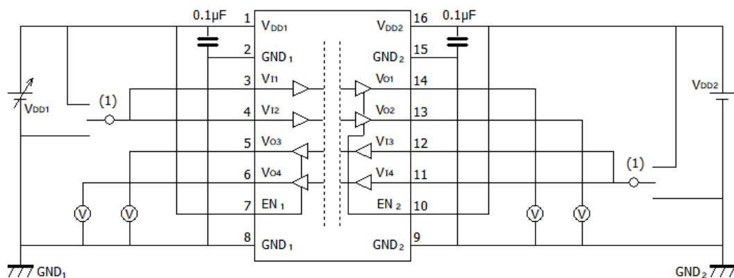
图 12.1.4. DCL542L01/DCL542H01 V_{DDIU+}/V_{DDIU-} 特性测定回路图
