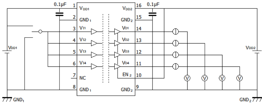
图 12.2.2. DCL540L01/DCL540H01 V_{OH}/V_{OL} 特性测定回路图
