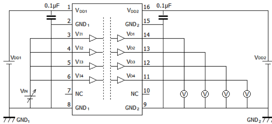
图 12.3.1. DCL540C01/DCL540D01 V_{IH}/V_{IL} 特性測定回路図
