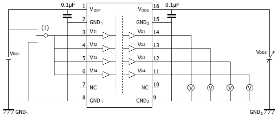
图 12.1.4. DCL540C01/DCL540D01 V DD2UV+ / V DD2UV- 特性测定回路图
