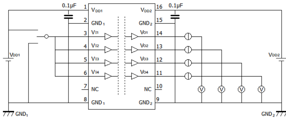
图 12.2.1. DCL540C01/DCL540D01 V_{OH}/V_{OL} 特性测定回路图
