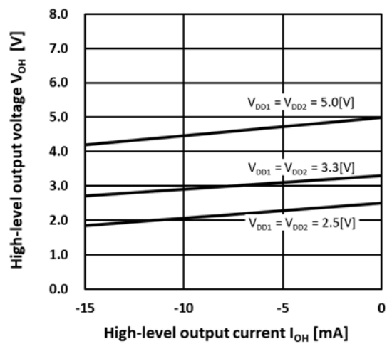
図 13.5. V_{OH}-I_{OH}
