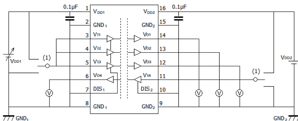
図 12.1.5. DCL541A01/DCL541B01 V_{DD1UV+} / V_{DD1UV-} 特性測定回路図
