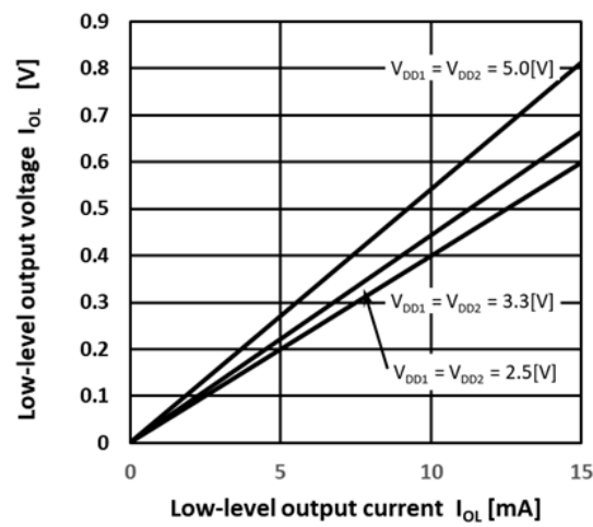
図 13.6. V_{OL}-I_{OL}
