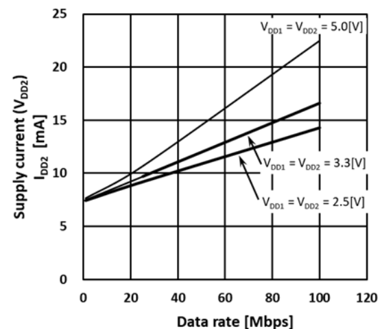
図 13.4. DCL541x01 I_{DD2} 動作電流—データレート
