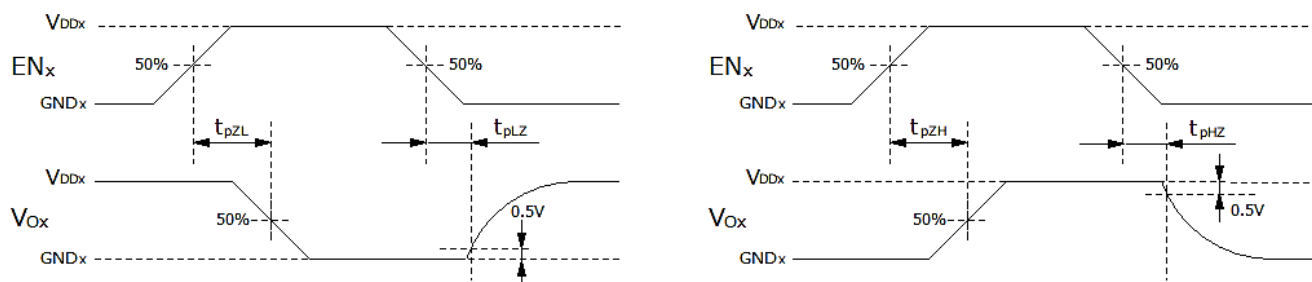
図 12.5.4. DCL54xL01/ DCL54xH01 イネーブル伝搬遅延時間波形図
