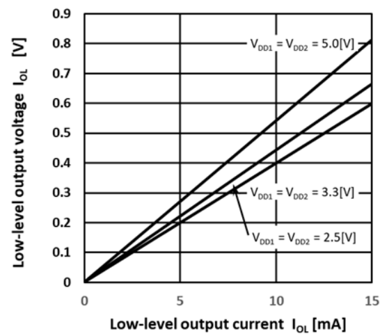
图 13.6. V_{OL}-I_{OL}
