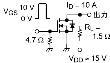
図 6.2.1 スwitching時間の測定回路例
