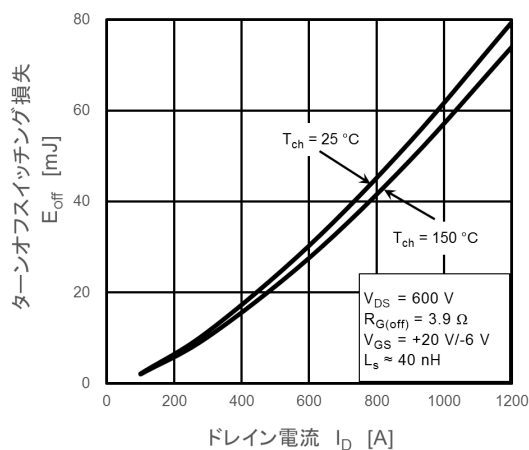
図 8.8 E_{off} - I_D
