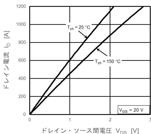
図 8.1 I_D - V_{DS} (注1)
