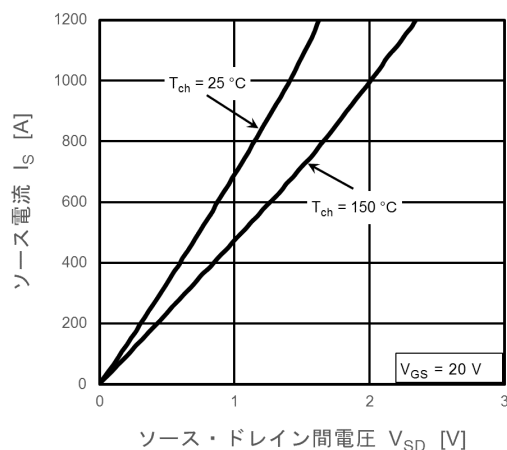
図 8.3 I_S - V_{SD} (注1)
