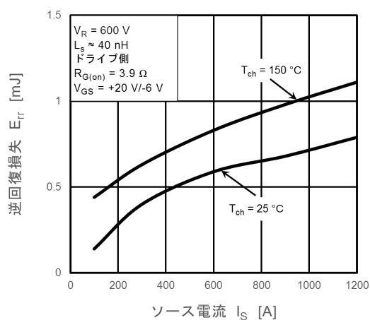
図 8.9 E_{rr} - I_S
