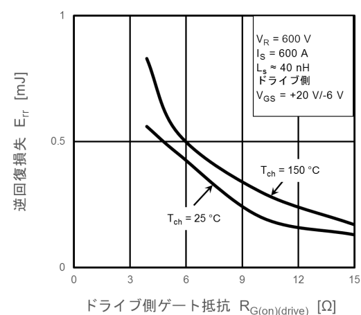
図 8.12 E_{rr} - R_{G(on)}
