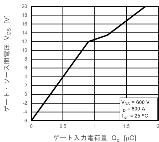
図 8.5 V_{GS} - Q_g
