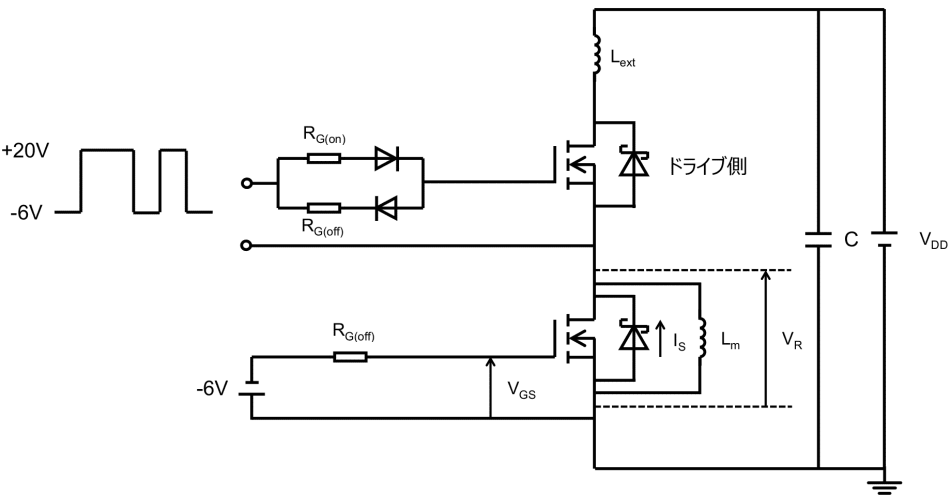
図 7.4 逆回復特性測定回路(ハイスайдスイッチング)
