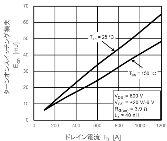
図 8.7 E_{on} - I_D
