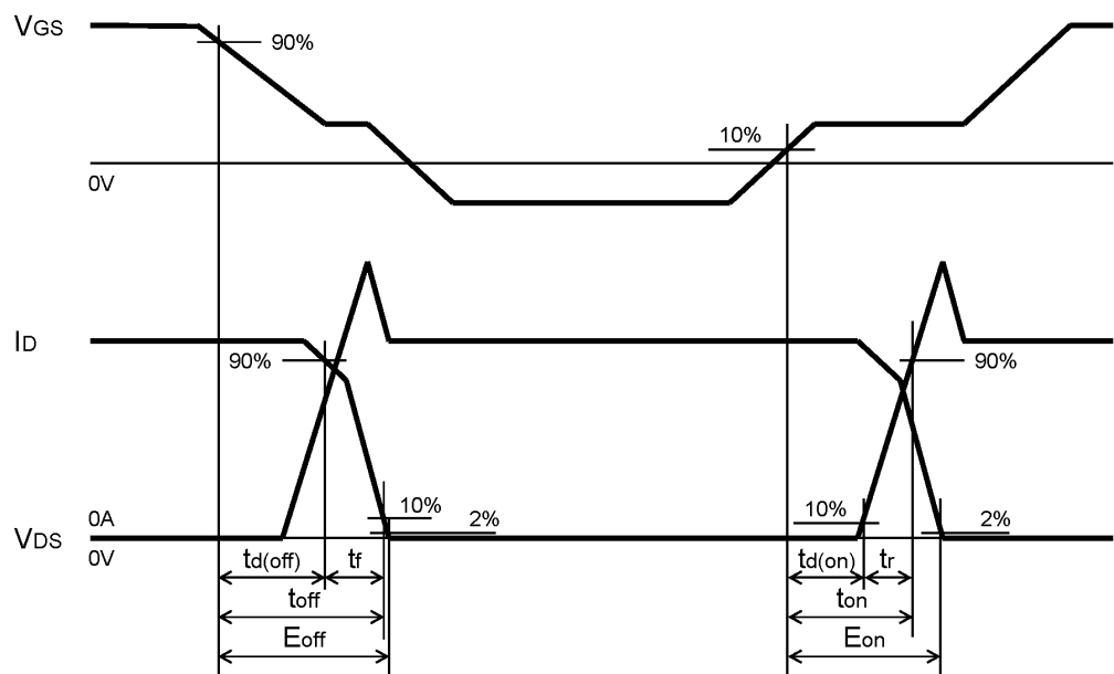
図 7.3 タイミングチャート(MOSFET部)
