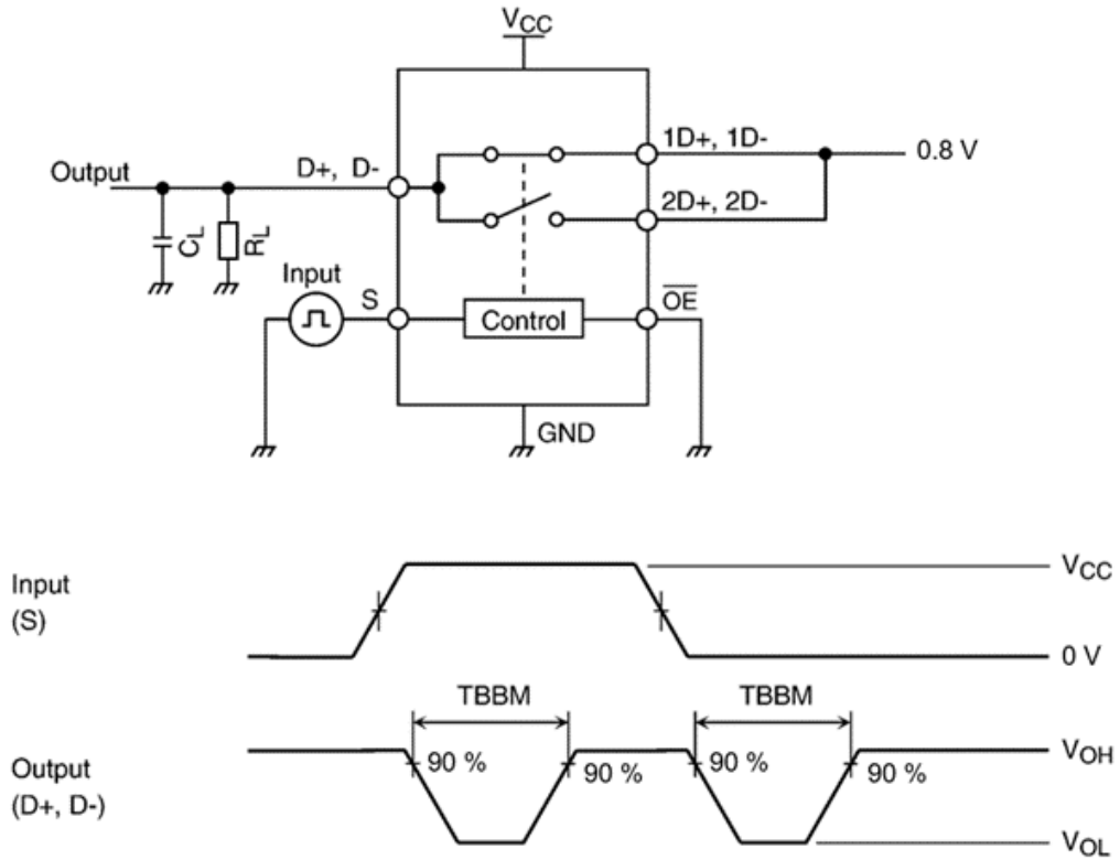
図 11.3 ブレーク・ビフォー・メーカー (TBBM)
