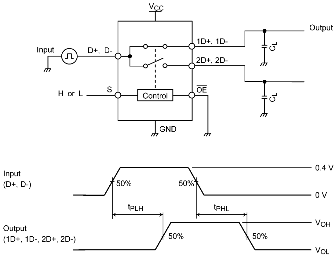
図 11.4 他遷移出力間スキュー ( t_{SK(P)} = |t_{PHL} - t_{PLH}| )
