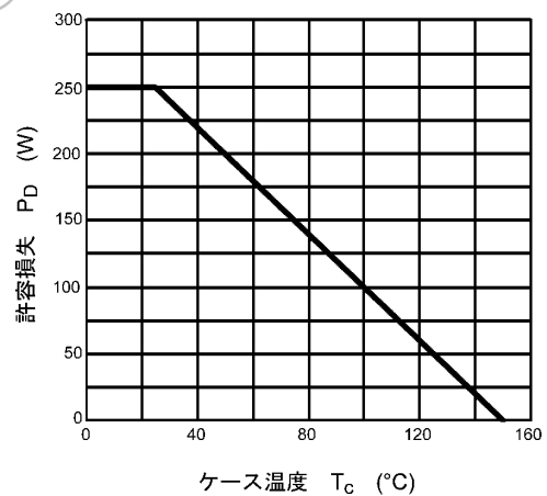
図 8.12 P_D - T_c (最大値 (保証値))
