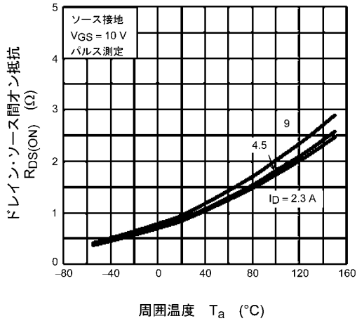
図 8.7 R_{DS(ON)} - T_a
