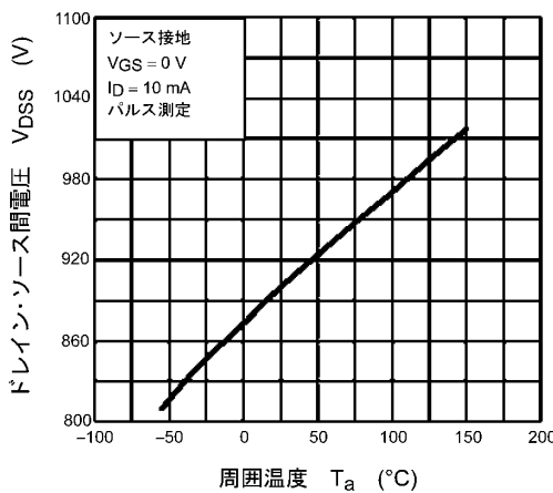
図 8.5 V_{DS} - T_a
