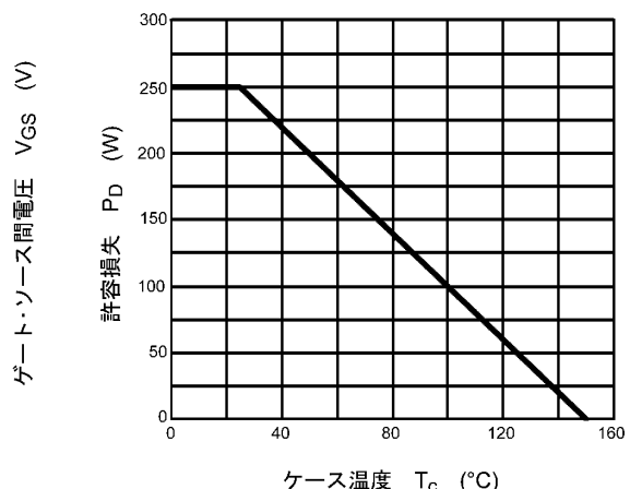
図 8.12 P_D - T_c (最大値 (保証値))
