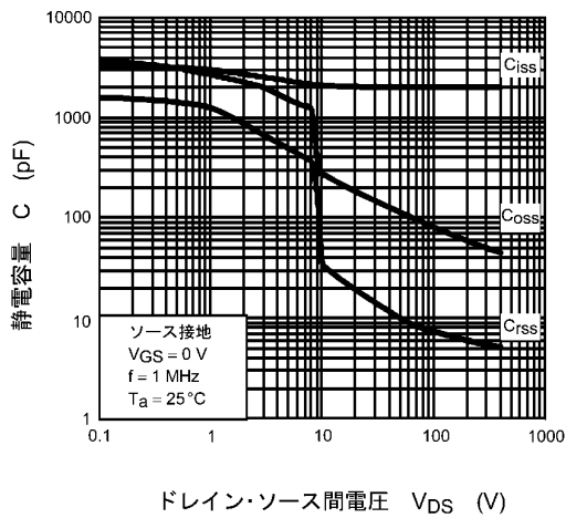
図 8.9 C - V_{DS}
