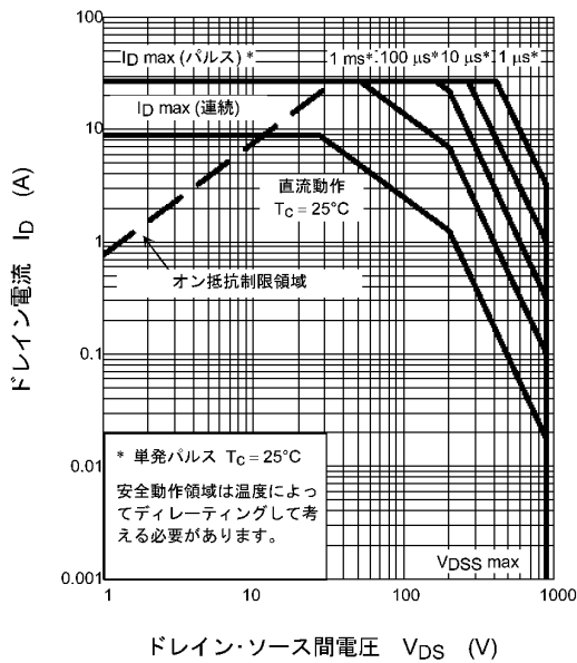
ドレイン・ソース間電圧 V_{DS} (V) 図 8.14 安全動作領域 (最大値 (保証値))
