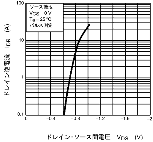
図 8.8 I_{DR} - V_{DS}
