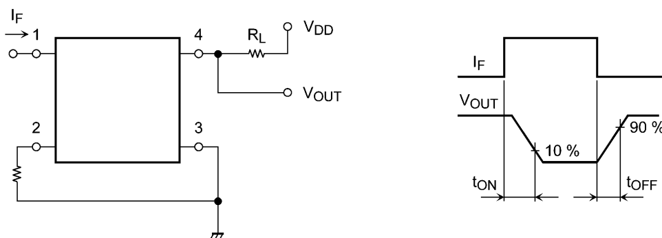
図 13.1 スwitching時間測定回路, 波形
