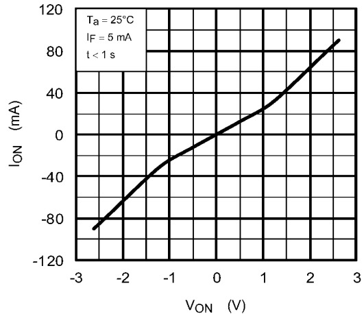
図 16.4 I_{ON} - V_{ON}
