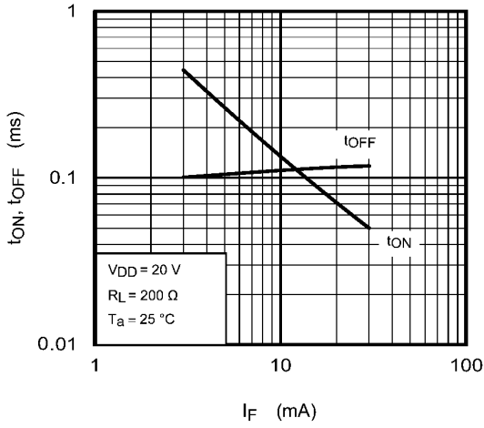
図 16.7 t_{ON}, t_{OFF} - I_F
