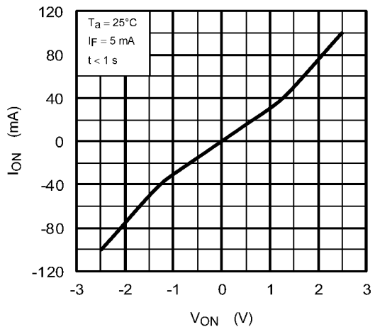
図 16.4 I_{ON} - V_{ON}
