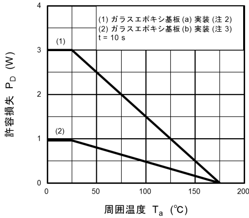
図 8.16 P_D - T_a (最大値 (保証値))
