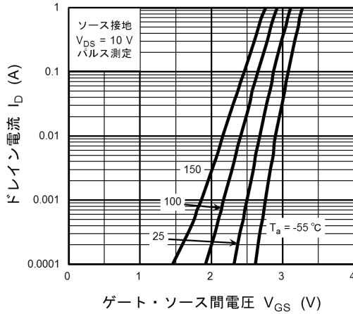
図 8.7 I_D - V_{GS}
