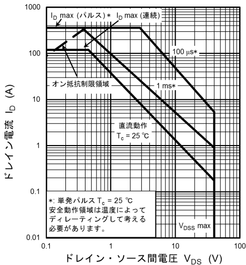
図 8.18 安全動作領域 (最大値 (保証値))
