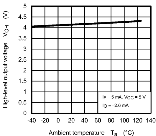
Fig. 12.2.5 V_{OH} - T_a
