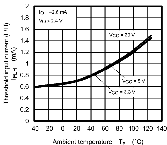
Fig. 12.2.11 I_{FLH} - T_a
