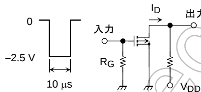
(a) 測定回路
