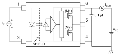
Fig. 12.1.5 I_{CCH} Test Circuit
