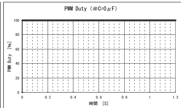
[SEL2=Low、コンデンサ値=0 \mu F]
