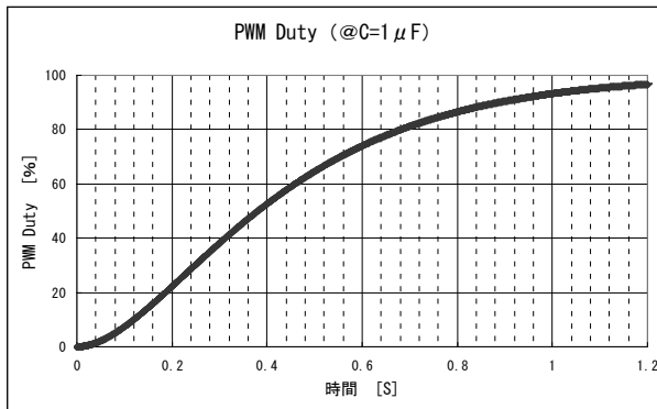
[SEL2=High、コンデンサ値=1 \mu F]
