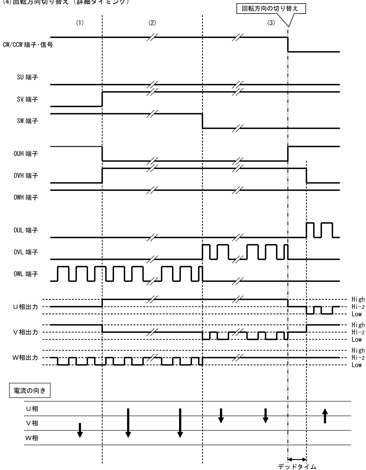
(4) 回転方向切り替え (詳細タイミング)
