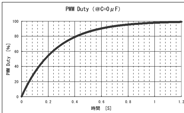
[SEL2=High、コンデンサ値=0 \mu F]
