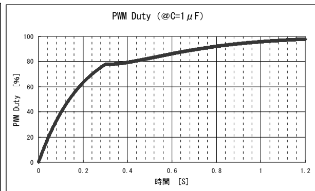
[SEL2=Low、コンデンサ値=1 \mu F]
