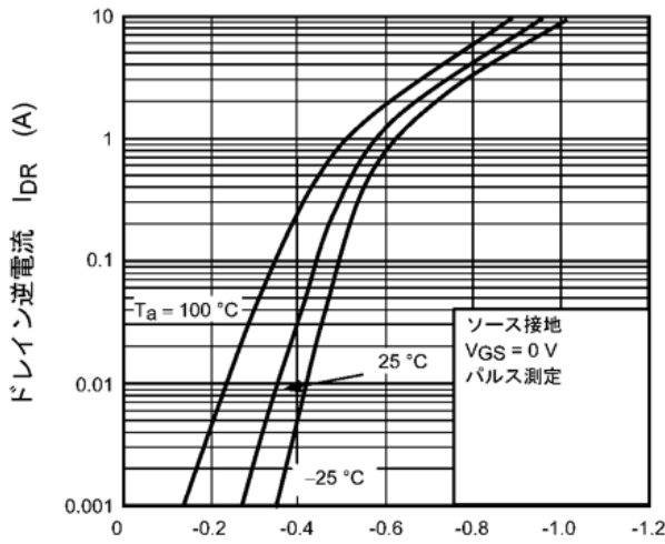
図 8.9 I_{DR} - V_{DS}
