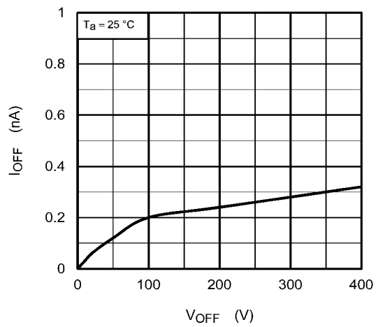
図 12.1.10 I_{OFF} - V_{OFF}
