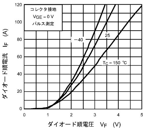
図 8.11 I_F - V_F
