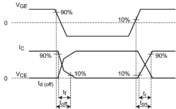
図 6.2.2 スwitching時間のタイミングチャート
