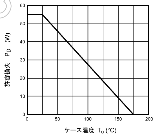
図 8.12 P_D - T_c (注7) (最大値 (保証値))
