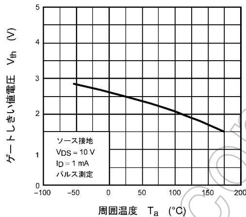
図 8.9 V_{th} - T_a (注7)
