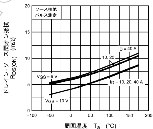
図 8.6 R_{DS(ON)} - T_a (注7)
