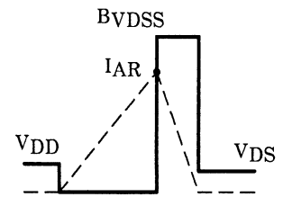
測定波形
