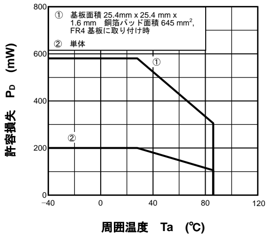
P D - T a (SMV)
