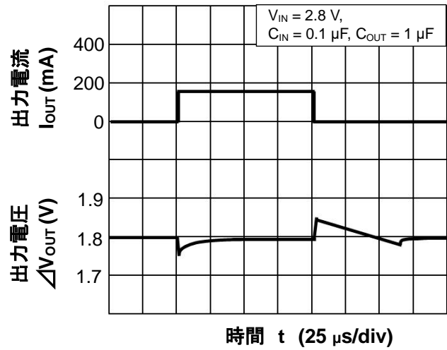
V_{OUT} = 1.8\text{ V} ( I_{OUT} = 1\text{ mA} \leftrightarrow 150\text{ mA} )
