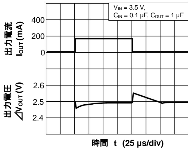
V_{OUT} = 2.5\text{ V} ( I_{OUT} = 1\text{ mA} \leftrightarrow 150\text{ mA} )
