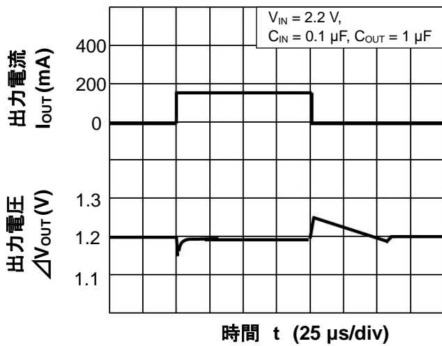
V_{OUT} = 1.2\text{ V} ( I_{OUT} = 1\text{ mA} \leftrightarrow 150\text{ mA} )
