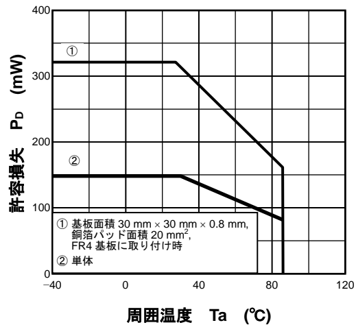
P D - T a (ESV)
