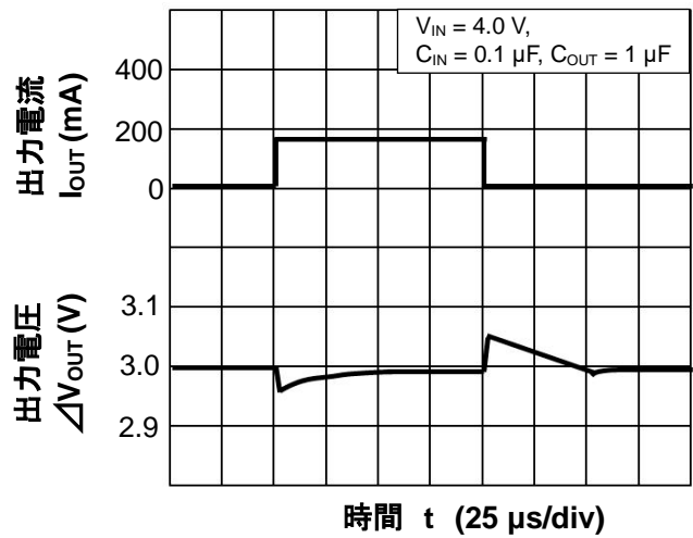
V_{OUT} = 3.0\text{ V} ( I_{OUT} = 1\text{ mA} \leftrightarrow 150\text{ mA} )
