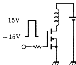
測定回路
