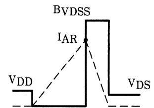
測定波形
